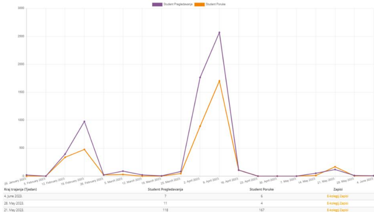
Slika 27. Statistika e-kolegija
