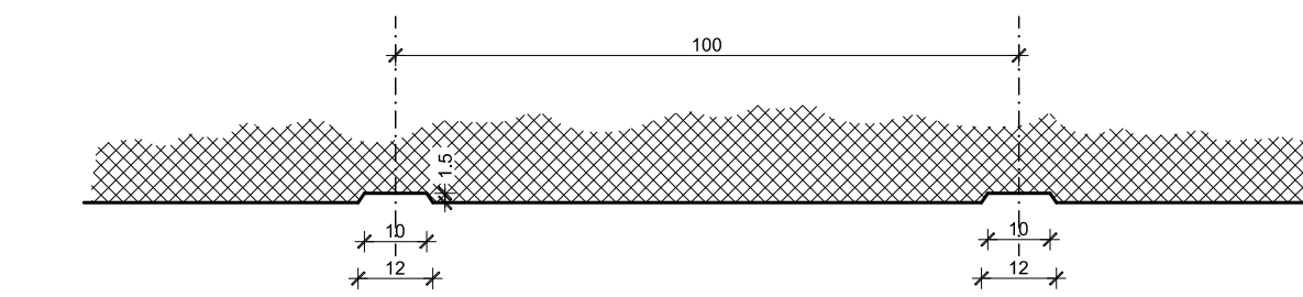
Detalj kanelura
