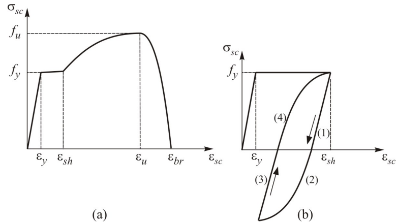
Crtež 5.4 Veza naprezanje-deformacija u čeliku za: (a) za monotono opterećenje; (b) cikličko opterećenje
