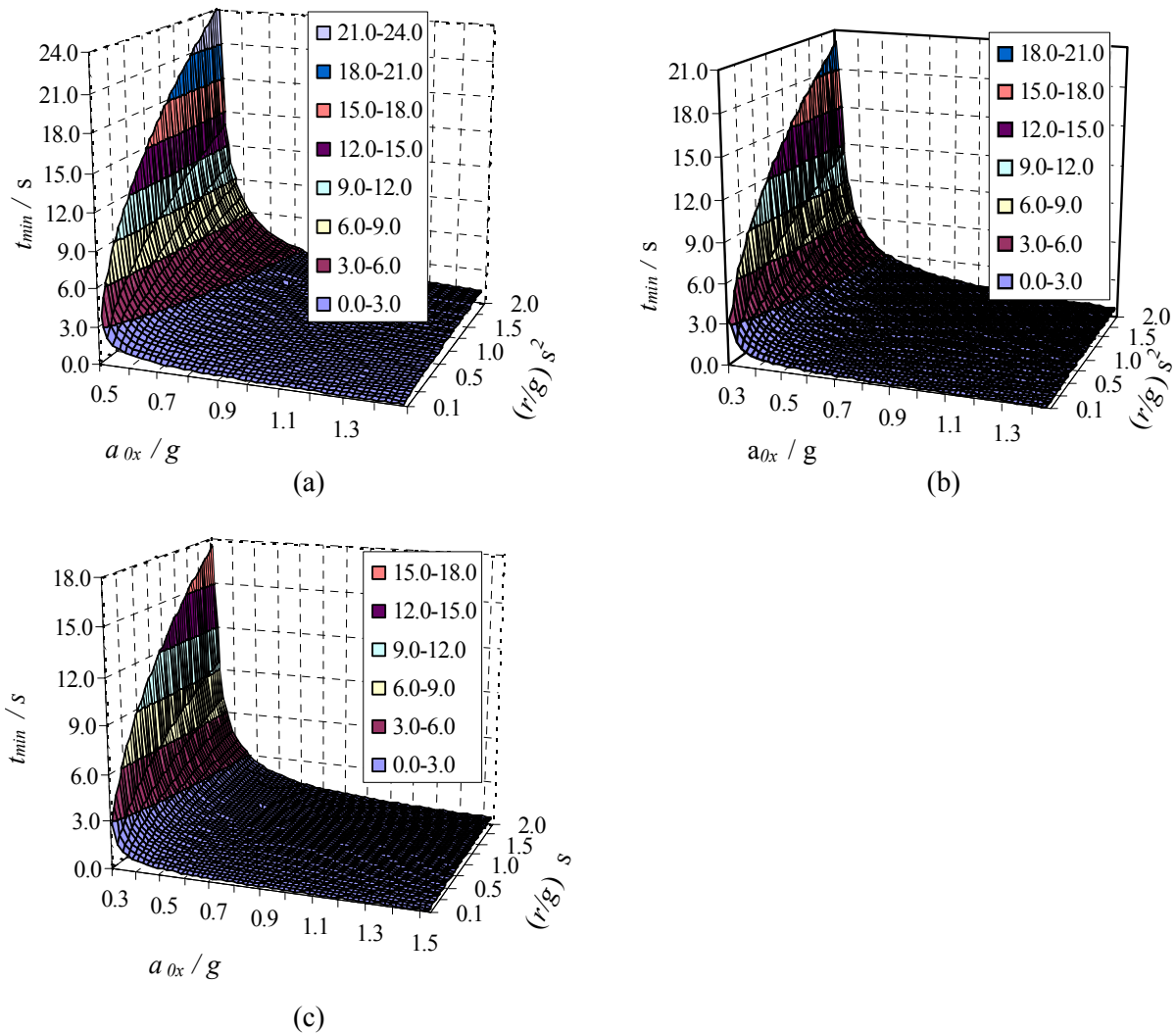
Crtež 4.29 Vrijednosti t_{\min} za: (a) h/l=2/1 ; (b) h/l=3/1 ; (c) h/l=4/1
