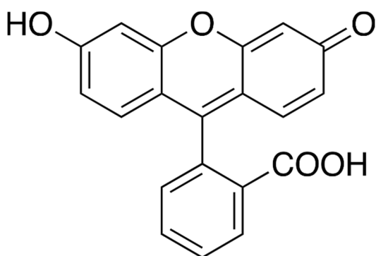
Slika 2. Struktura fluoresceina [34]
