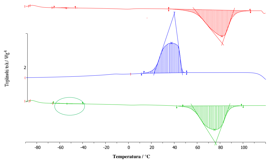
Slika 38. DSC krivulje uzorka PEO/10 % PEG-POSS (1. mjerenje)
