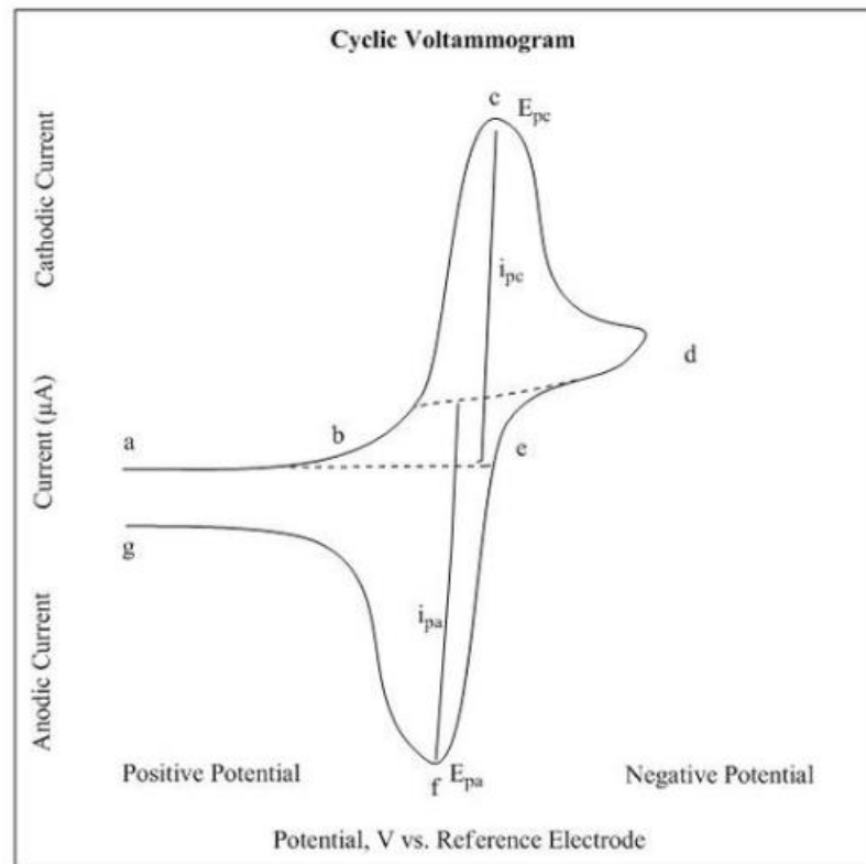
Slika 6. Ciklički voltamogram
