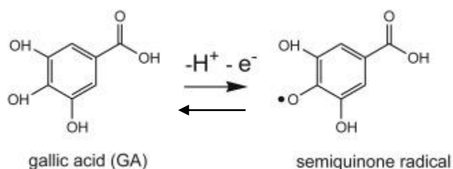
Slika 20. Oksidacija galne kiseline u semikinon radikal
