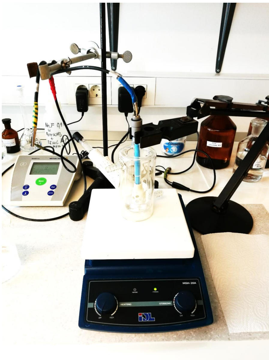
Slika 3. Uređaj za potenciometrijska određivanja
