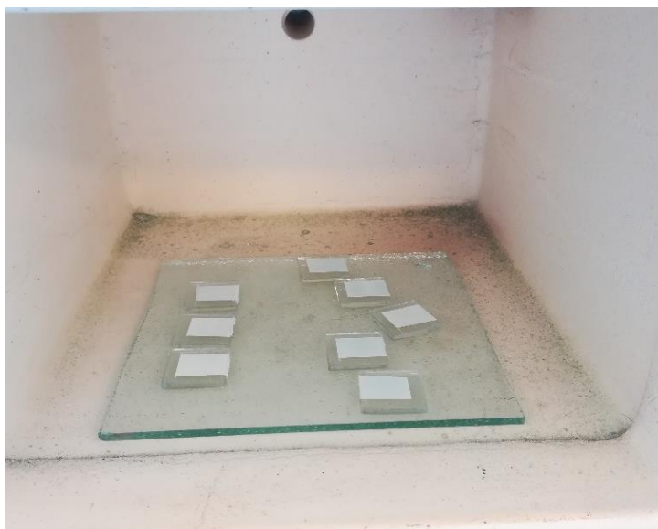
Slika 25. Pečenje oksidnog sloja u laboratorijskoj peći
