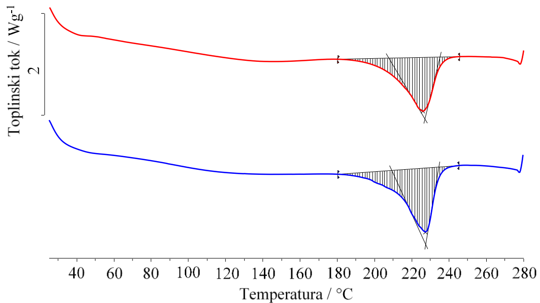
Slika 35. Usporedba normaliziranih DSC krivulja (prvo zagrijavanje) uzoraka izvornog (crveno) i sintetiziranog (plavo) PVAL-a
