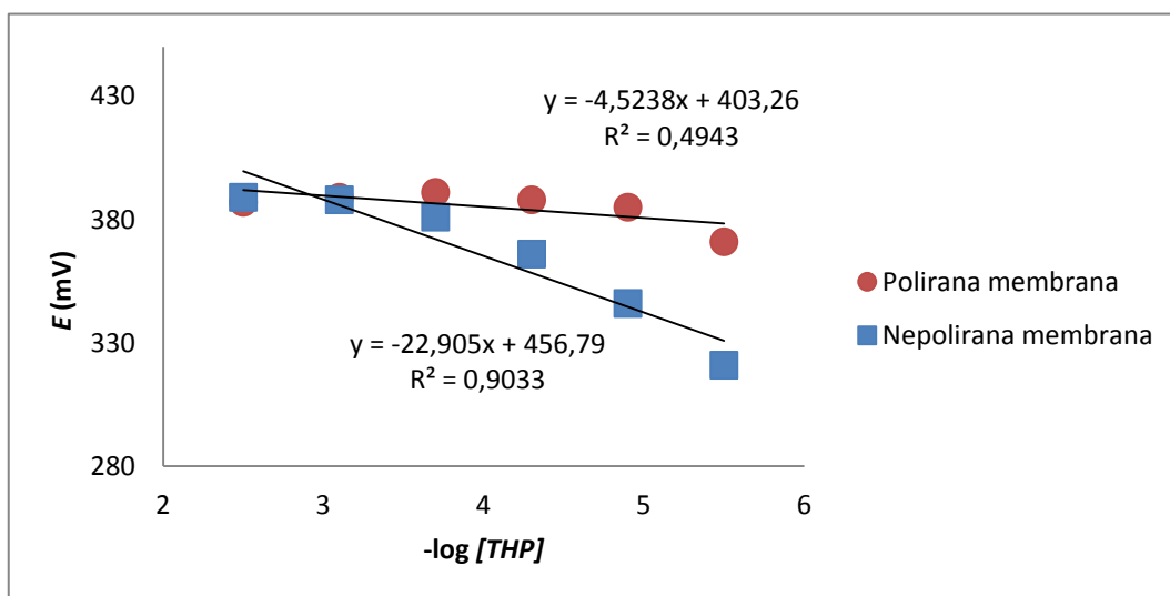
Slika 9. Ovisnost promjene potencijala elektrode s membranom 1 o koncentraciji THPHCl. Koncentracijsko područje je od 3,16 \cdot 10^{-6} do 3,16 \cdot 10^{-3} M, a pH = 4,5
