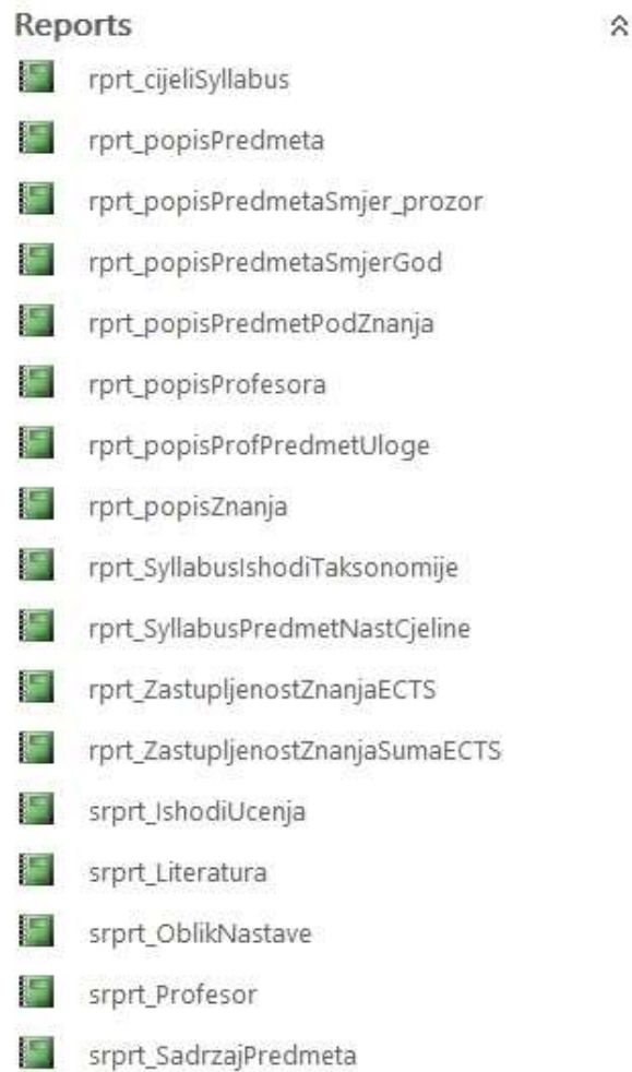
Slika 41 - popis izvješća
