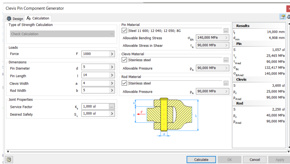
Slika 5.5 - Proračun klina [12]
