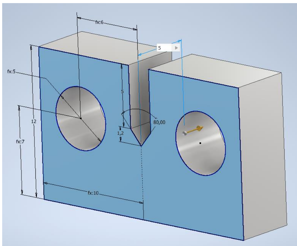
Slika 5.2- Dimenzije epruvete [12]
