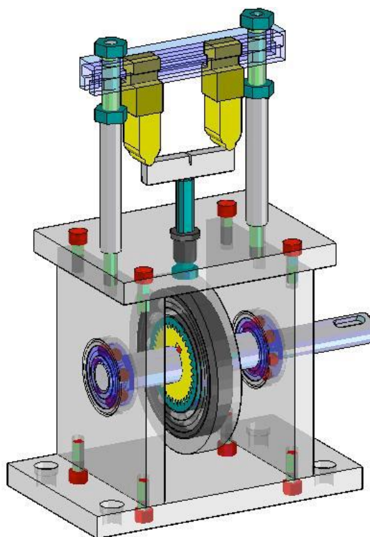
Slika 1.4 - Uređaj za generiranje pukotine [6]
