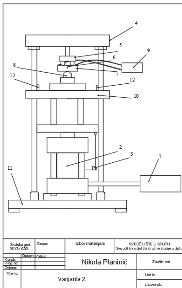
Slika 2.5 - Varijanta 2
