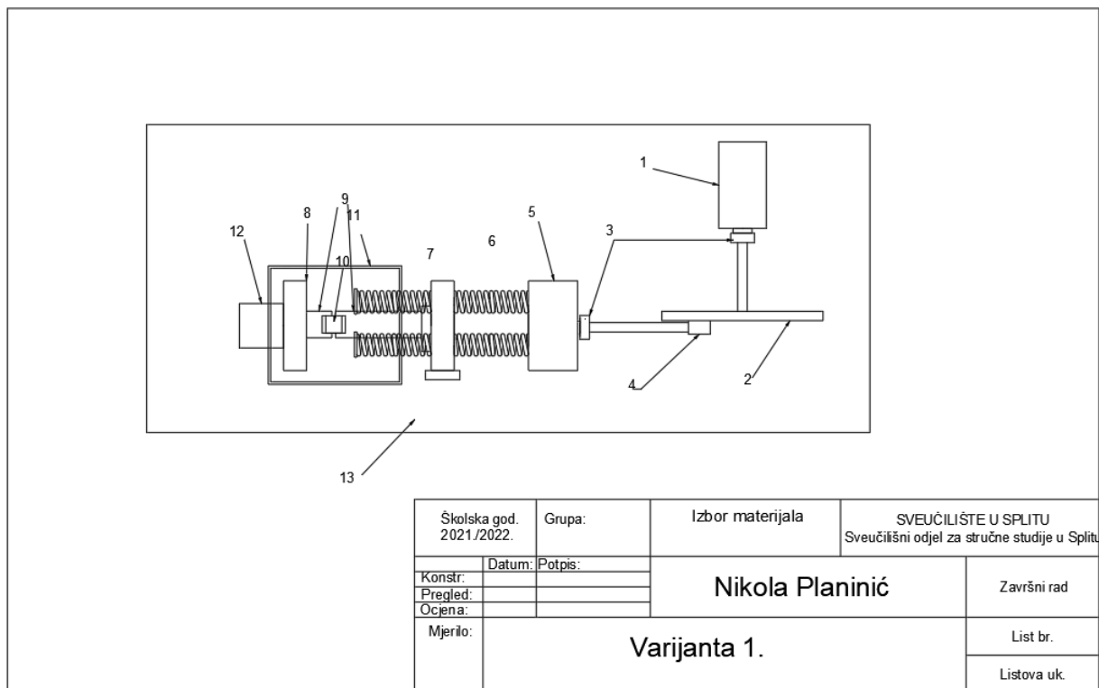
Slika 2.4 - Varijanta 1
