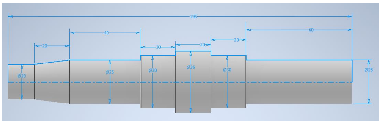
Slika 5.14 - Vratilo [12]
