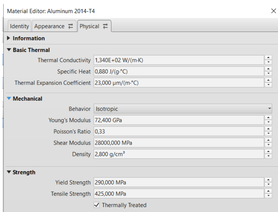
Slika 5.1- Odabrani materijal [12]
