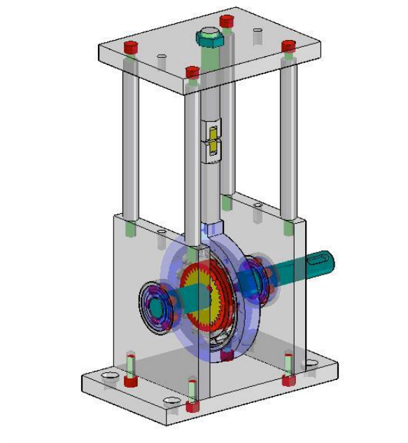
Slika 1.6 - Shema uređaja za generiranje pukotine epruvete za vlačno opterećenje [6]
