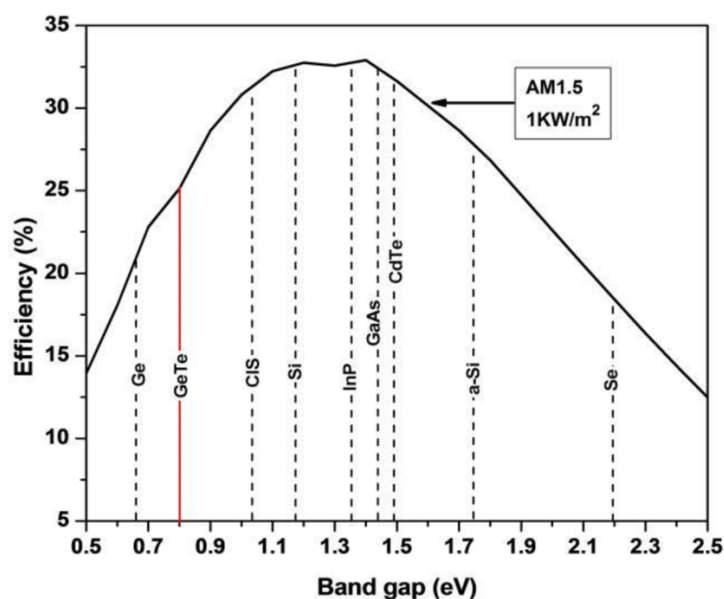
Slika 11. Maksimalna teorijska djelotvornost ćelije u ovisnosti o širini zabranjene vrpce [10]
