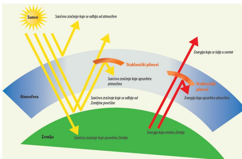
Slika 3. Ozračenje u slojevima atmosfere [4]
