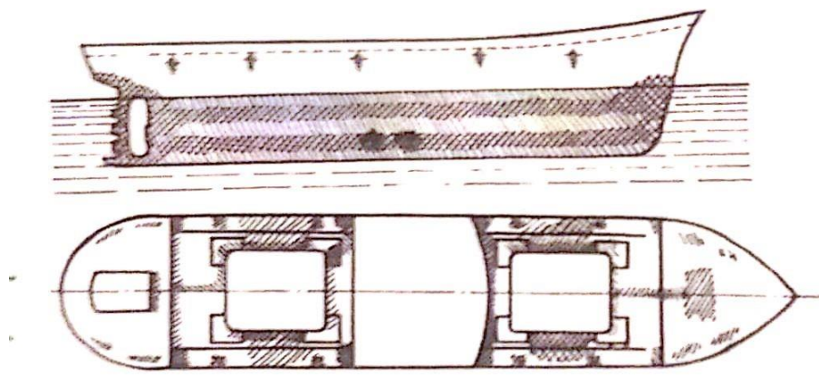
Slika 4. Prikaz intenziteta oštećenja podvodne brodske oplate i vanjske palube s obzirom na osobitosti konstrukcije u uvjeta eksploatacije
