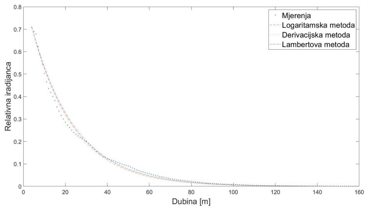
Slika 4.16 Izmjerena i procijenjena vrijednost 10. profila za težinsku postepenu metodu.
