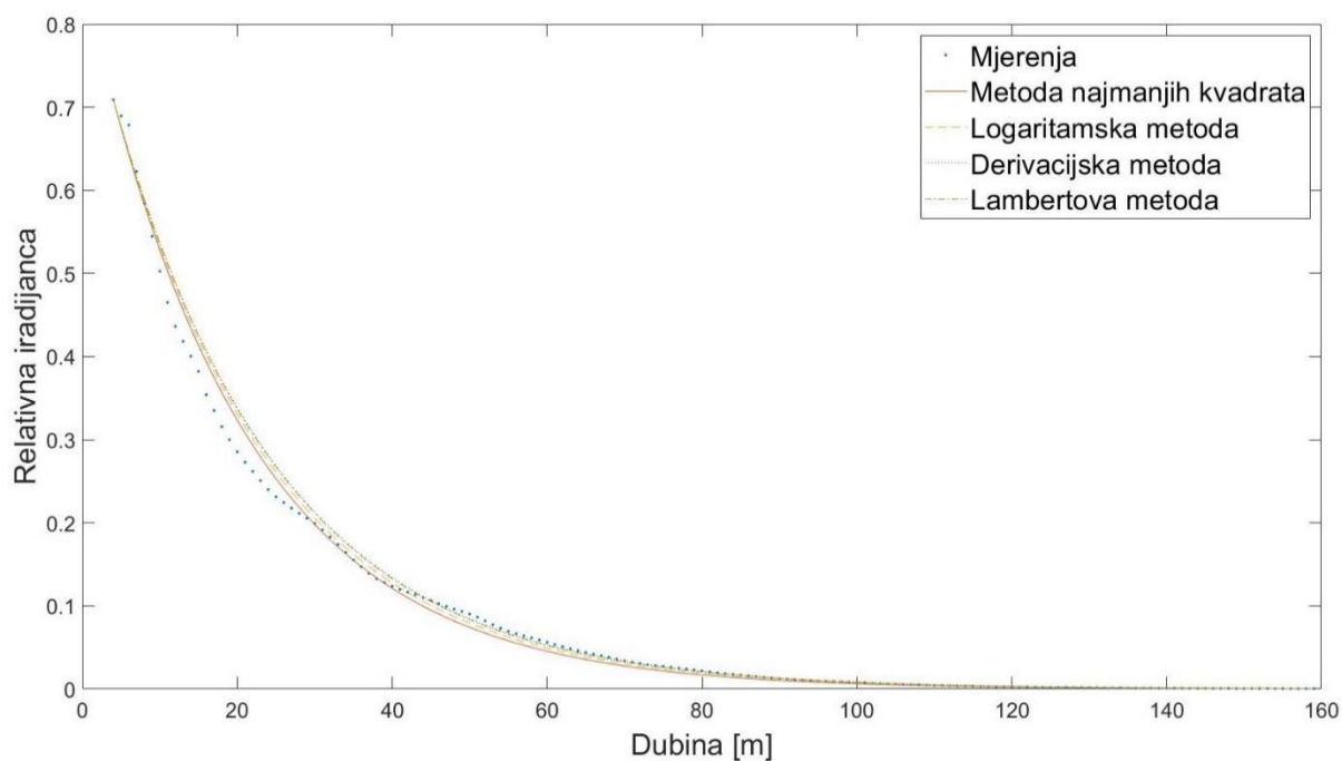
Slika 4.14 Izmjerena i procijenjena vrijednost 10. profila za običnu postupenu metodu.
