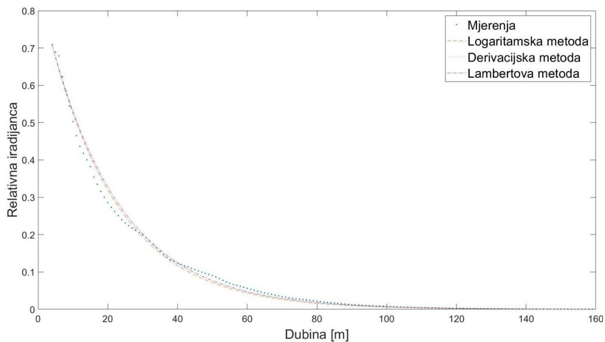
Slika 4.15 Izmjerena i procijenjena vrijednost 10. profila za težinsku direktnu metodu.
