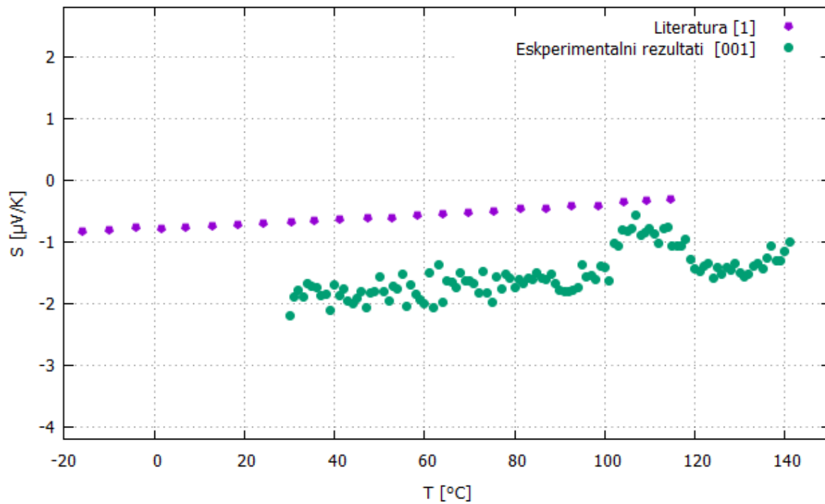
Slika 33. Rezultati mjerenja temperaturene ovisnosti Seebeckovog koeficijenta u intervalu [35 °C, 140 °C] za kristalografski smjer [001] uzorka GaPd 2 . (Preuzeto iz (pog. Prilog 1))
