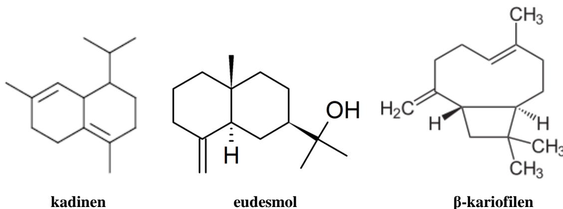
Slika 23. Biciklički seskviterpeni
