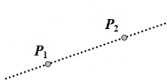
Tablica 3. Aksiomi origamija
