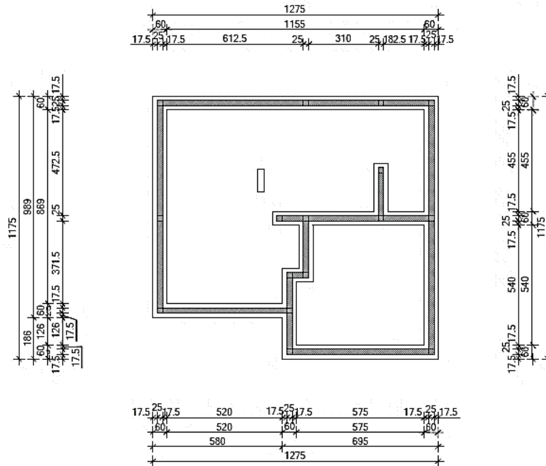
Slika 18. Tlocrt temelja
