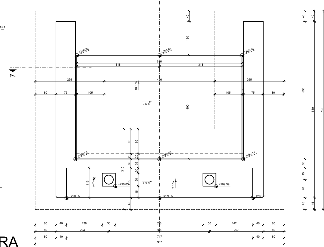
PLAN OPLATE UPORNJAKA U1 1:50
