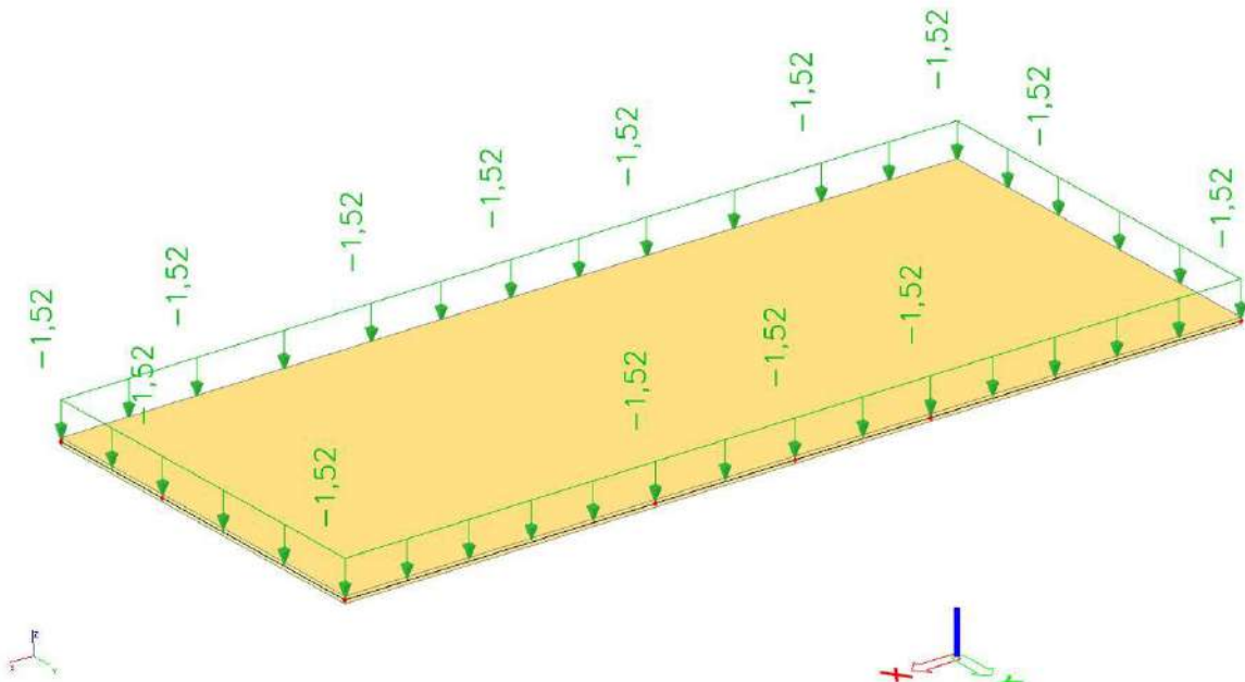
Slika 3.1.1 Dodatno stalno djelovanje G_1 [ \text{kN/m}^2 ]
