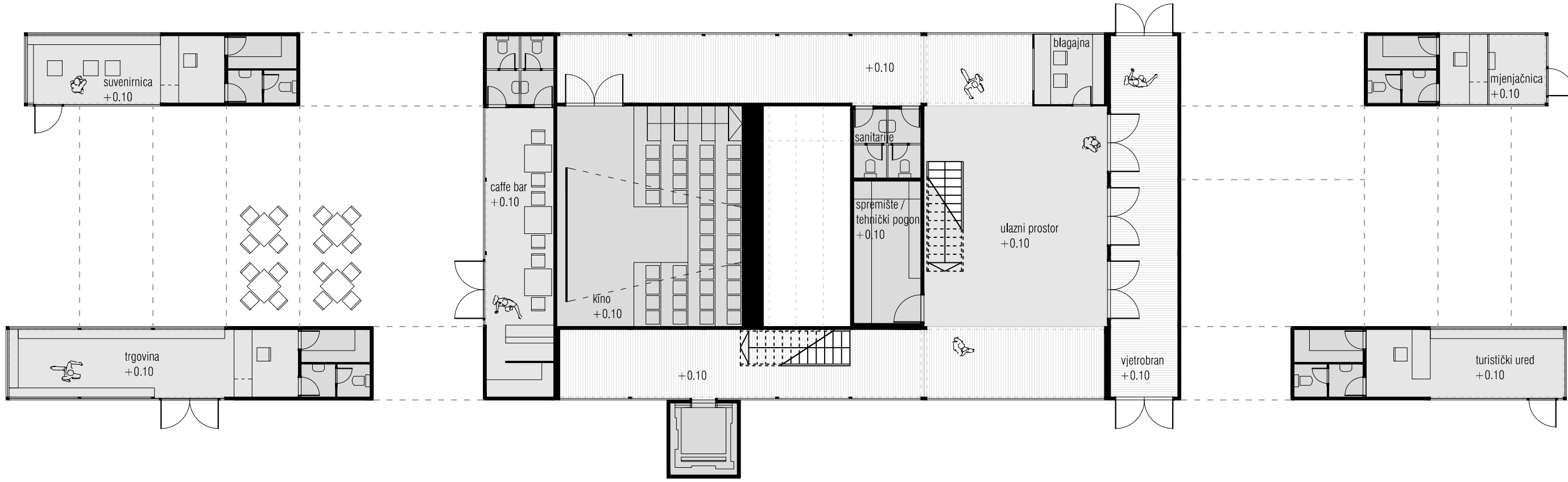
tlocrt prizemlja
