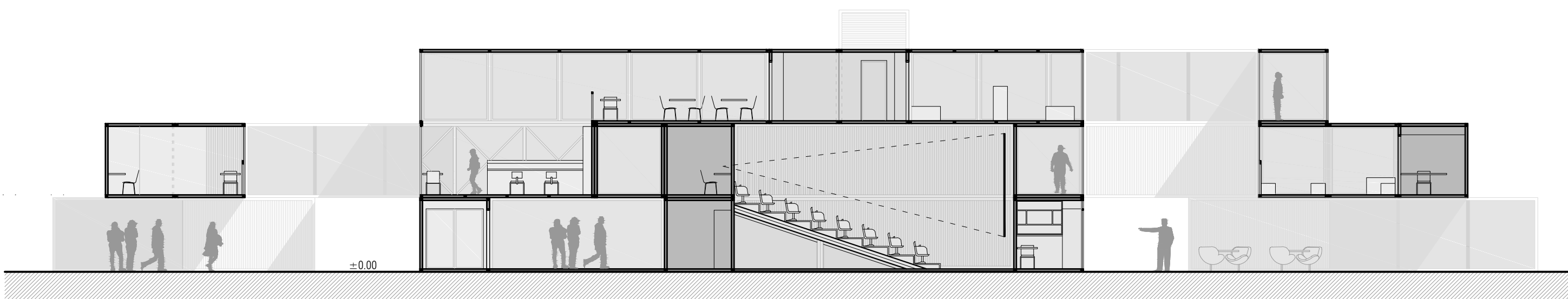
presjek
