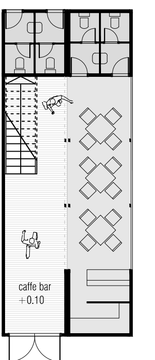
tlocrt prizemlja
