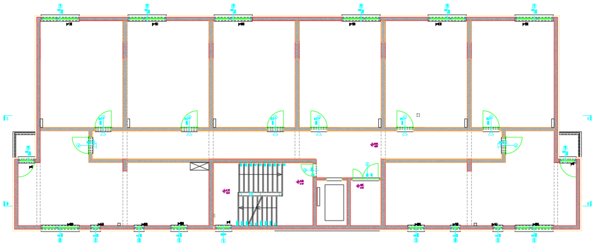
Slika 1.6. Tlocrt 2. kata
