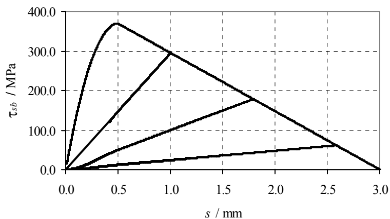
Crtež 5.22 Veza posmičnog naprezanja i posmičnih pomaka u trnu za slučaj cikličkog opterećenja
