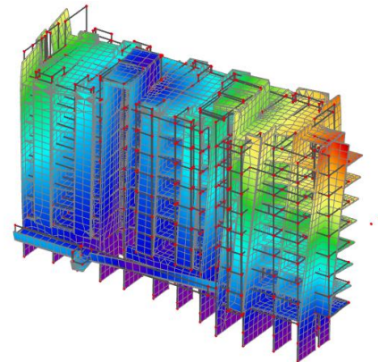
Slika 10.8 Drugi vlastiti vektor od djelovanja potresa na konstrukciju
