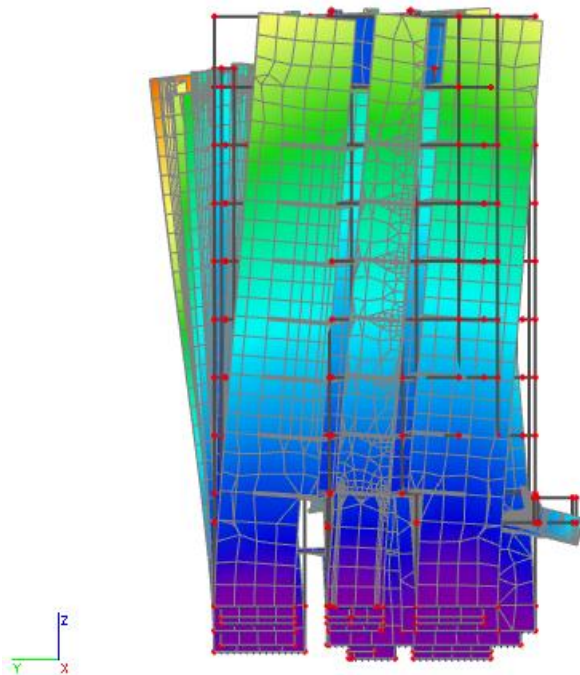
Slika 10.8 Drugi vlastiti vektor od djelovanja potresa na konstrukciju
