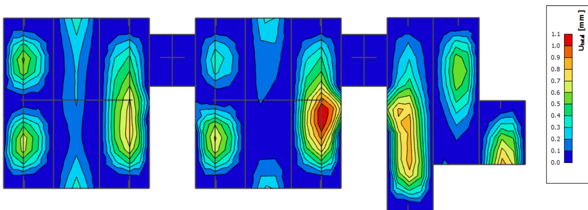
Slika 11.92 Prikaz progiba - GSU
