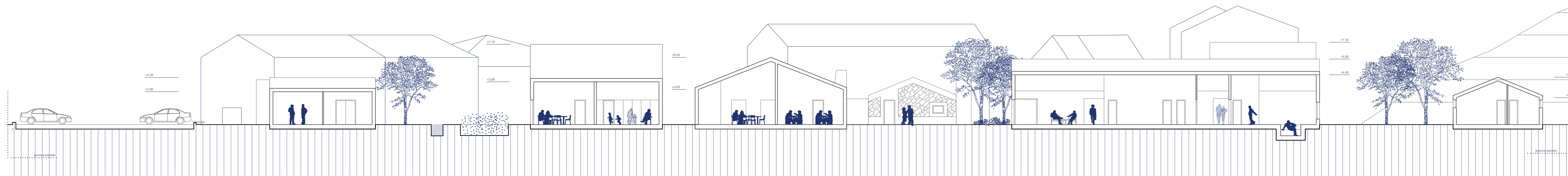
PRESJEK 1-1
