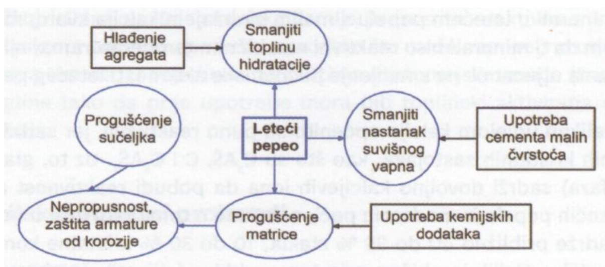
Slika 2.3.1. Djelovanje letećeg pepela na svojstva betona [1]
