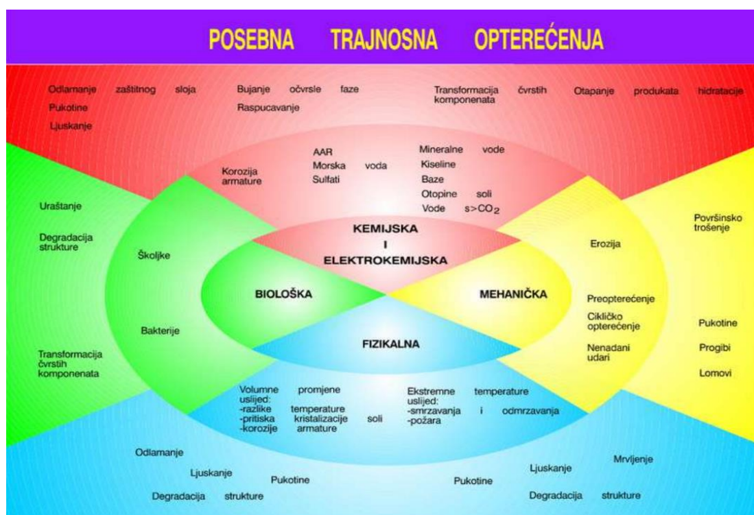
Slika 2.4. Trajnosna opterećenja [10]
