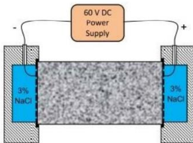
Slika 4.3. Uređaj za ispitivanje uzoraka na prolaz klorida [15]
