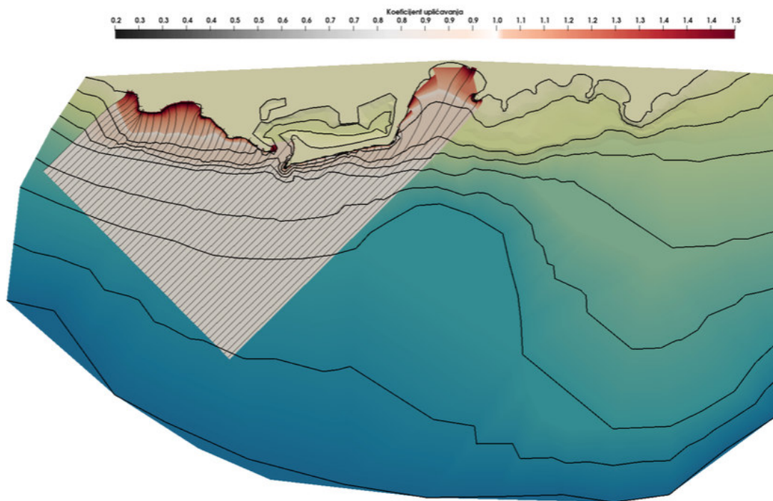
Slika 5.3.4. Utjecaj uplićavanja za sektor II ( H_s = 3,52m, T = 6s ) za petogodišnji val
