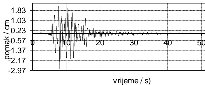
Slika 38. Vršno ubrzanje a_g = 0.10 g za Petrovac
