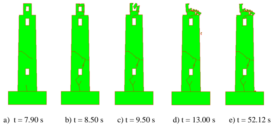
Slika 131. Širenje i nastanak pukotina za vršno ubrzanje \mathbf{a}_g = 1.85 \text{ g} za South Iceland
