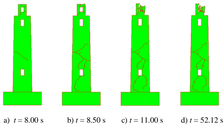
Slika 132. Širenje i nastanak pukotina za vršno ubrzanje \mathbf{a}_g = 1.90 \text{ g} za South Iceland
