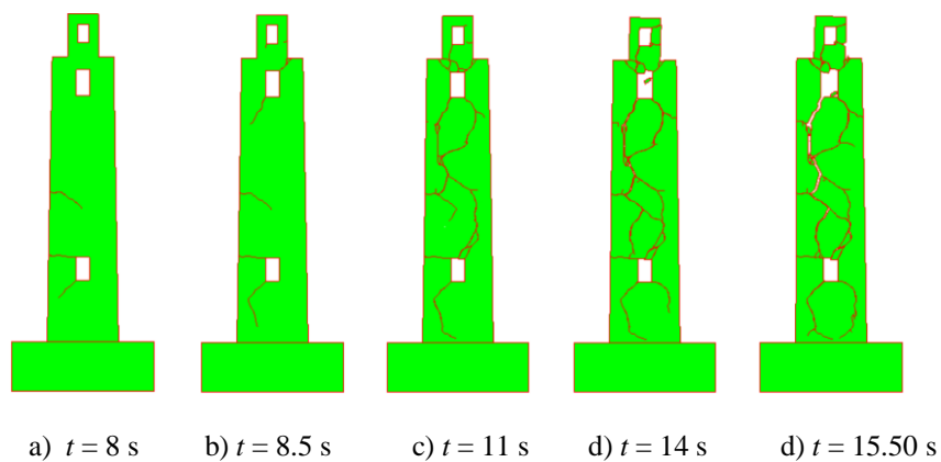
Slika 133. Širenje i nastanak pukotina za vršno ubrzanje \mathbf{a}_g = 1.95 \text{ g} za South Iceland
