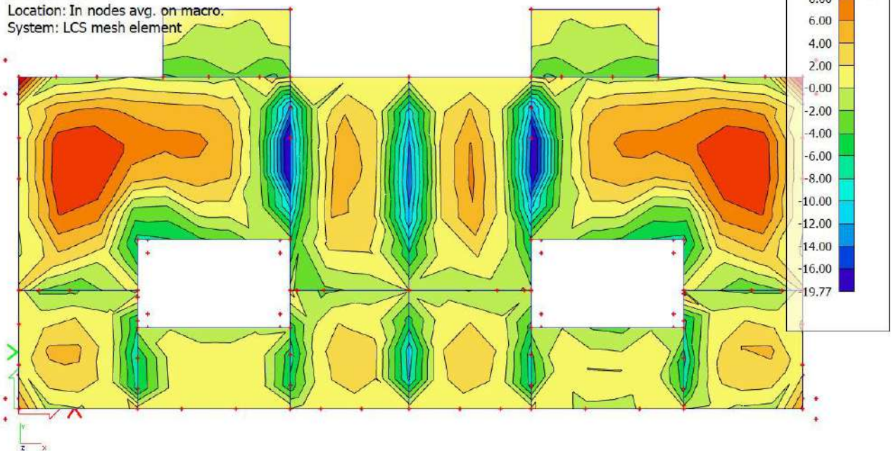
Slika 5.2 Moment savijanja M_{Ed,x} (kNm/m) za GSN-1
