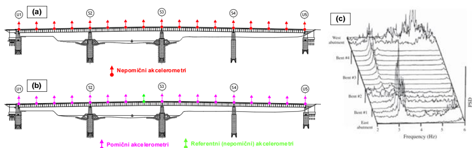
Slika 3. Položaj akcelometara za operacionu modalnu analizu. (a) Istovremeno mjerenje na više mjernih mjesta, (b) Višestruko mjerenje akceleracije na različitim mjernim mjestima na konstrukciji, (c) Primjer metode odabiranja vrha (eng. Peak – Picking method ) [9]
