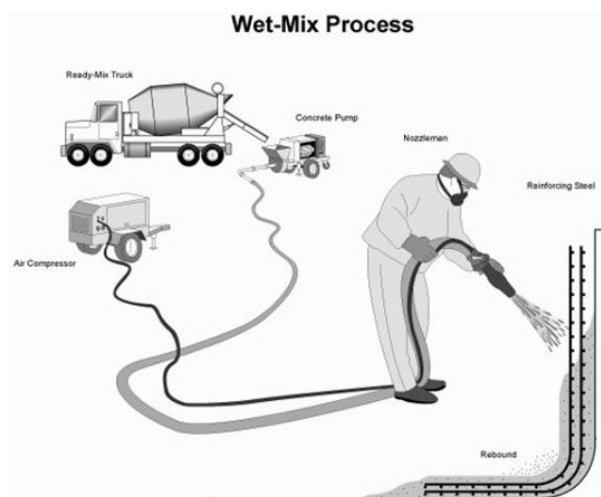
Slika 21. Mokri postupak
