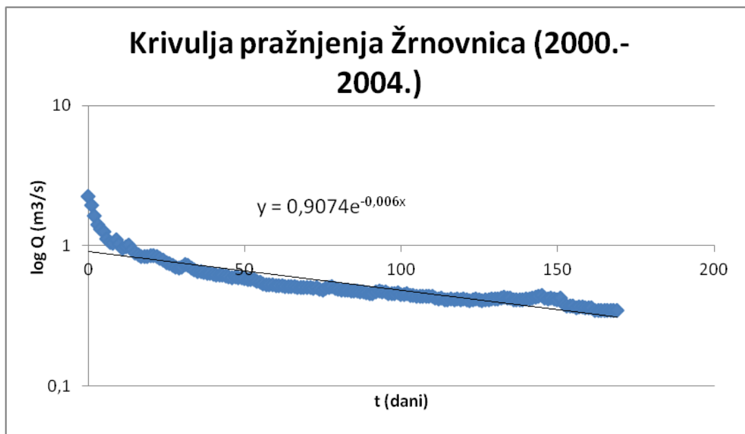
Slika 5.44. Krivulja pražnjenja rijeke Žrnovnice i njena jednađba
