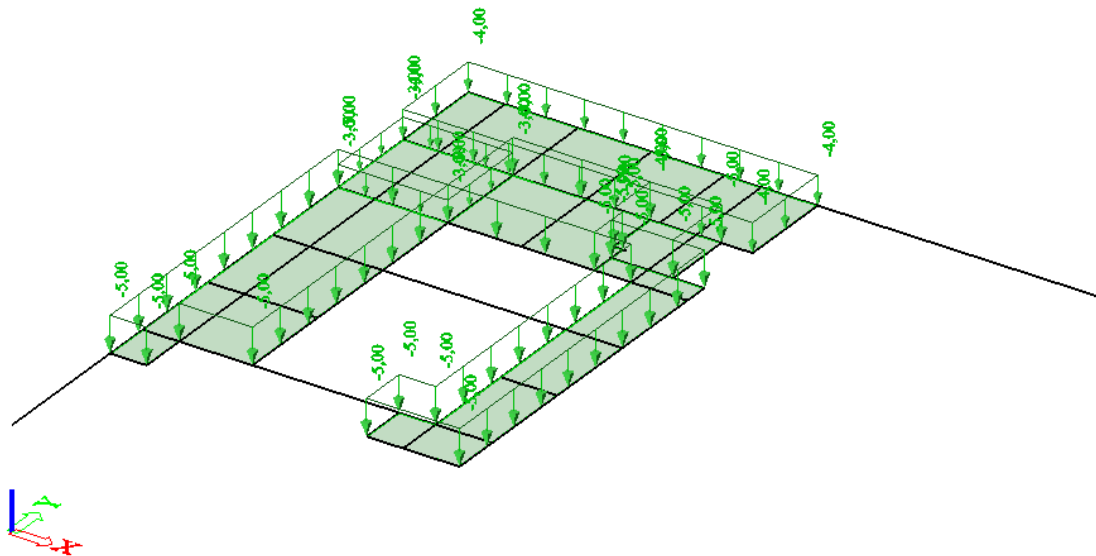
Slika 3.10. Prikaz raspodjele pokretnog opterećenja - pozicija 300
