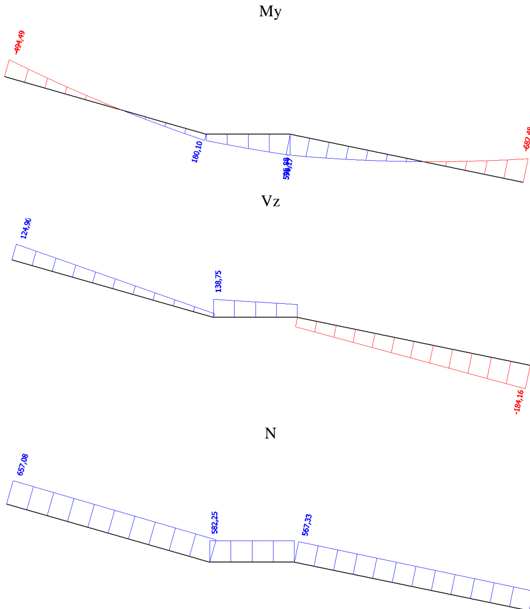
Slika 15.2. Prikaz reznih sila glavnog nosača stubišta
