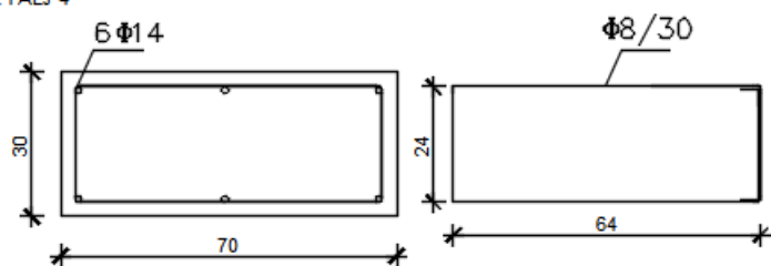
DETALJ 4
