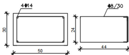
DETALJ 5
