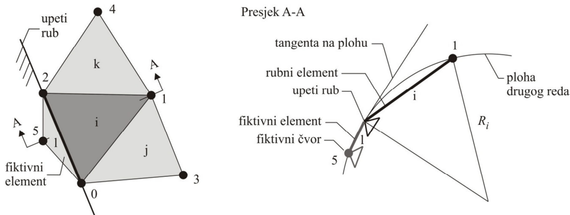
Crtež 5.10 Određivanje zakrivljenosti konačnog elementa i , u početnoj konfiguraciji za slučaj upetih rubnih uvjeta
