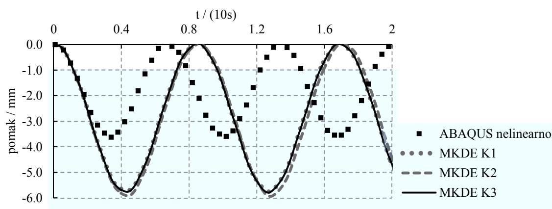
Crtež 5.17 Pomak središta kružne ploče za slobodno osciliranje – model I
