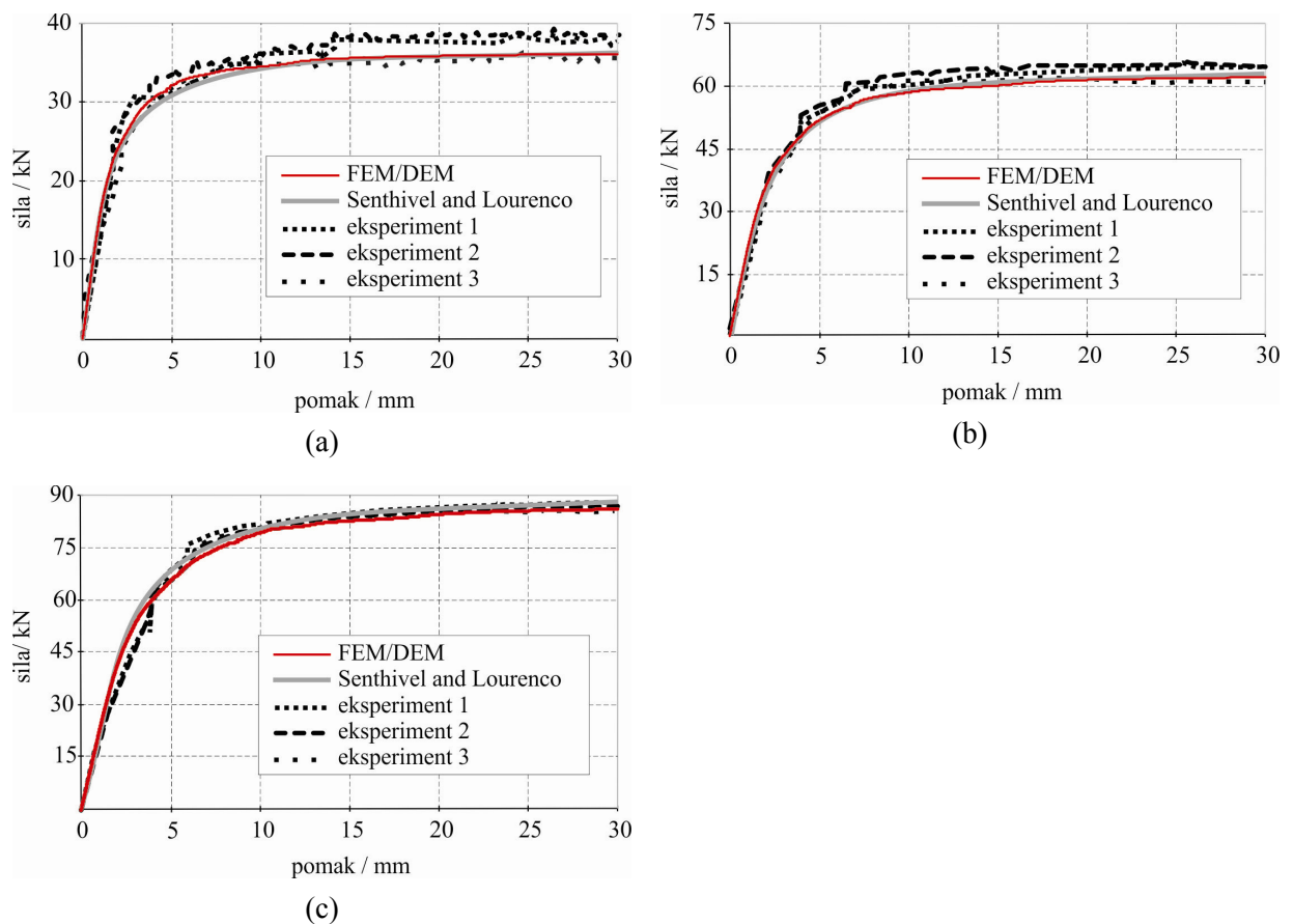
Crtež 4.12 Dijagrami sila pomak za predtlačna naprezanja od: (a) 0.5 MPa; (b) 0.875 MPa; (c) 1.25 MPa
