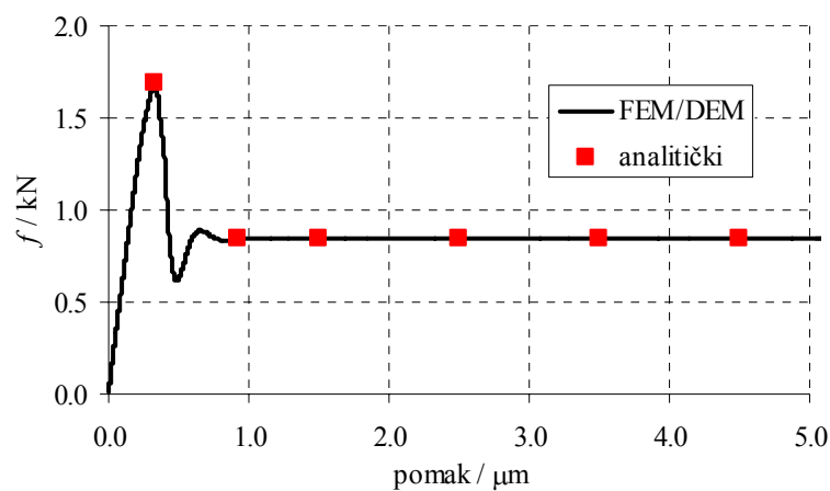
Crtež 3.21 Usporedba sile trenja u tijeku vremena dobivena analitički i numerički
