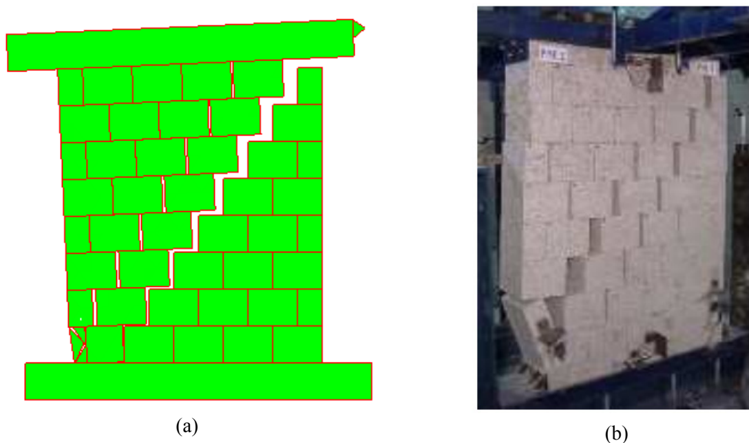
Slika 4.2 Oblik loma kamenog zida za predtlačno naprezanje 0.875 MPa: (a) numerički (b) eksperiment
