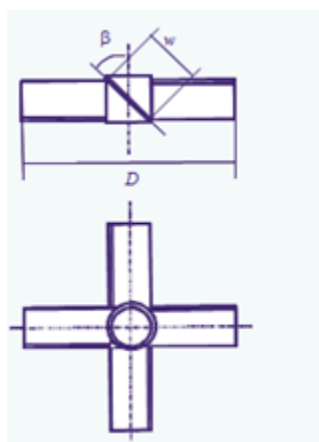
Slika 16. PBT miješalo
