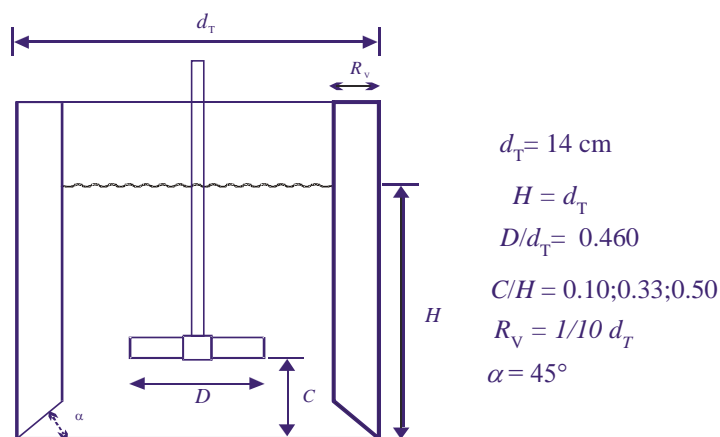
Slika 15. Kotlasti reaktor
