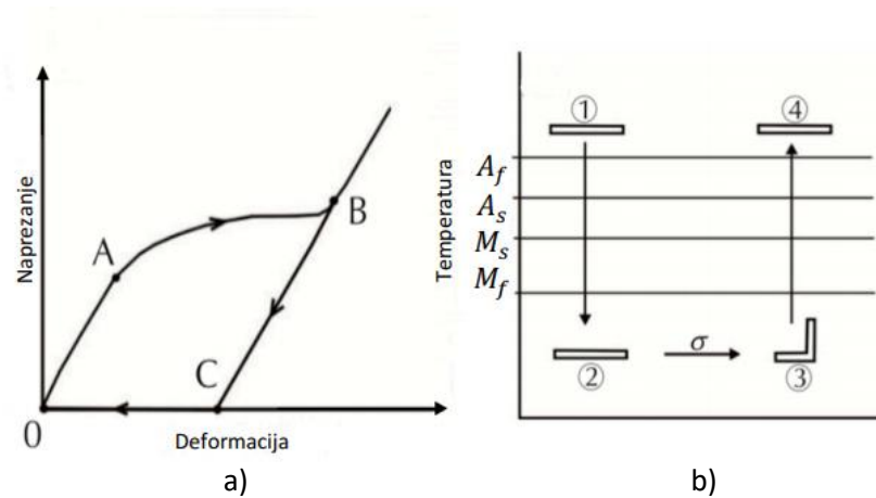
Slika 7. Prikaz dijagrama napreznja-deformacija za leguru s prisjetljivosti oblika (a) i shematski prikaz dijagrama jednosmjernog efekta prisjetljivosti oblika (b) (19)
