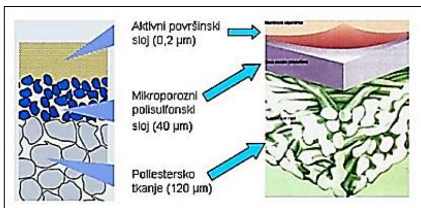
Slika 13. Sastav membrane. 20
