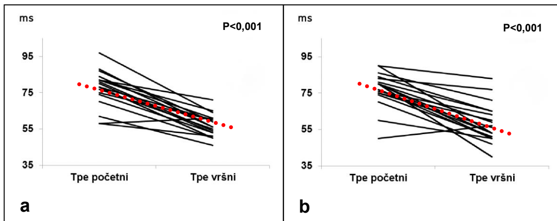
Slika 19. Vrijednosti Tpe intervala, u (a) kontrolnoj i (b) intervencijskoj skupini ispitanika, u mirovanju i vršnom opterećenju, 30. dana istraživanja.
