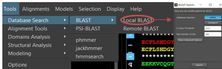
Slika 36. BLAST pretraživanje
