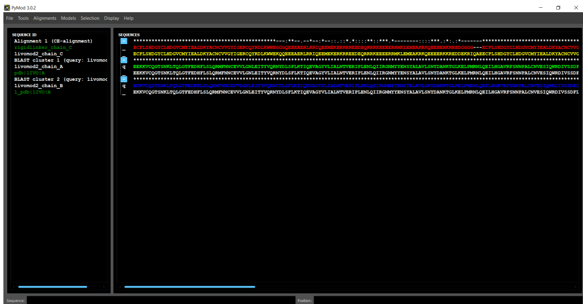
Slika 46. PyMod 3 alignm-i
