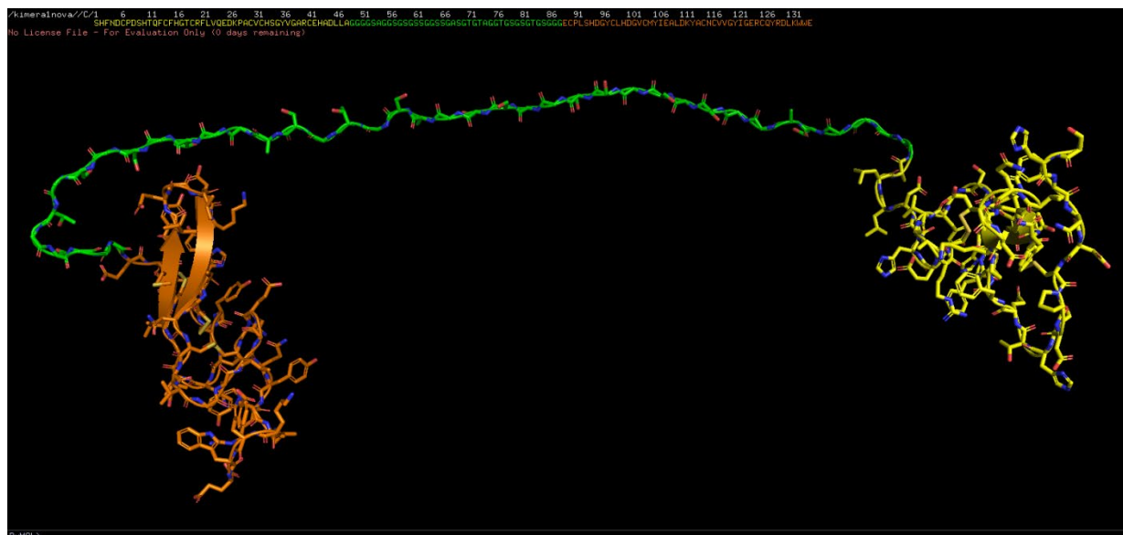
Slika 59. Struktura Kimere 5
