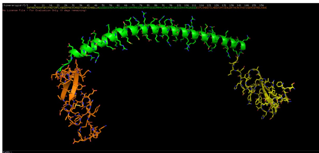
Slika 62. Struktura Kimere 6
