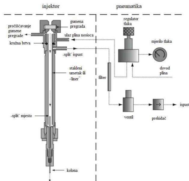
Slika 1.4. Schematski prikaz poprečnog presjeka split/splitless injektora (8).
