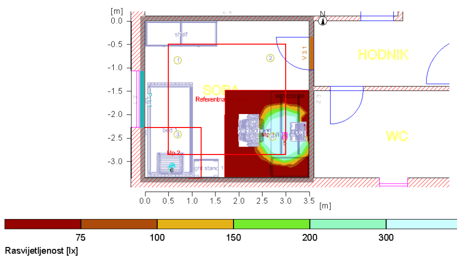
Slika 3.24. Rasvjetljenost radnog stola
