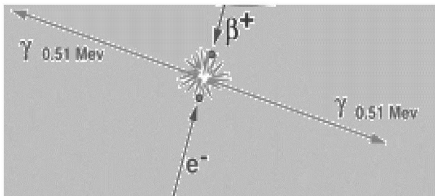
Slika 1. Anihilacijsko zračenje
