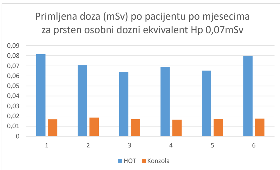
Grafikon 1. Usporedba primljene doze po jednom pacijentu za radna mjesta radiološkog tehnologa u HOT laboratoriju i radiološkog tehnologa za konzolom PET/CT uređaja mjereno prsten dozimetrom Hp 0,07mSv
