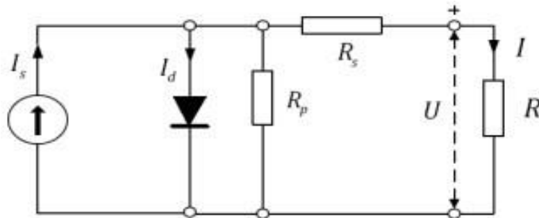
Slika 7. Ekvivalentni sklop sunčane ćelije [1]
