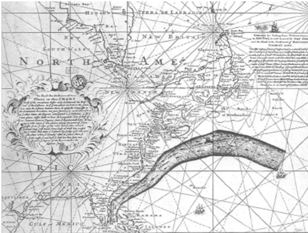
Slika 1. Franklinova i Folgerova karta Golfske struje [1]
