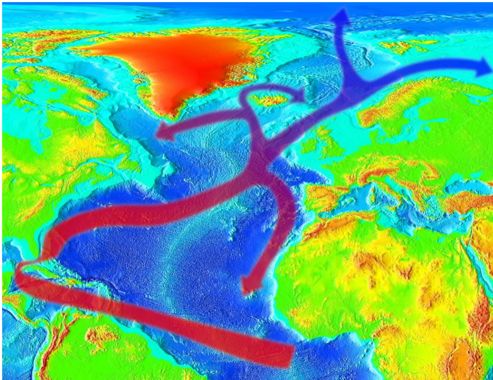
Slika 11. Smjer Sjevernoatlantske struje[4]
