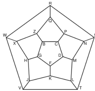
Slika 2.1: Ikozijska igra
