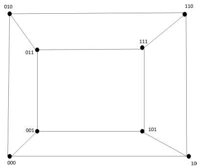
Slika 1.10: Q_3
