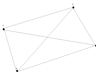
Slika 1.7: K_4
