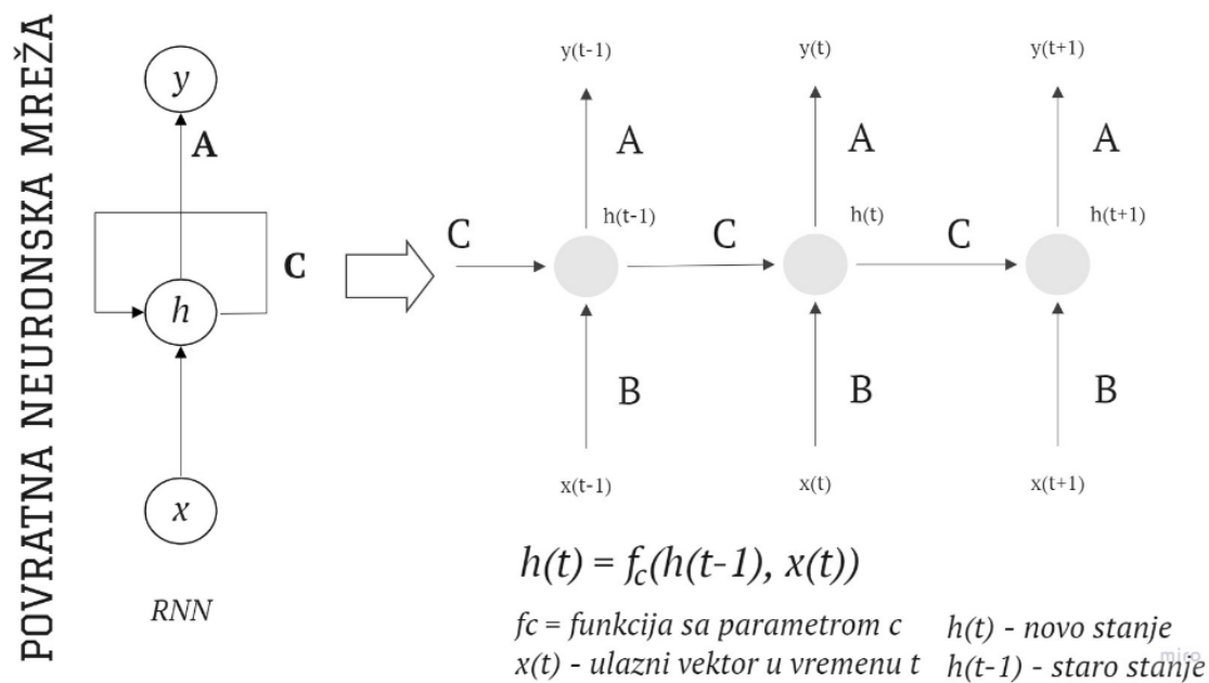
Slika 10 RNN model
