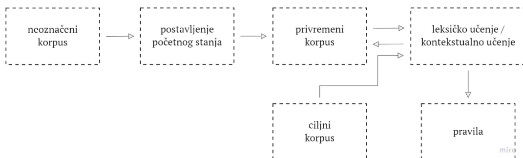
Slika 3 Brillov označivač
