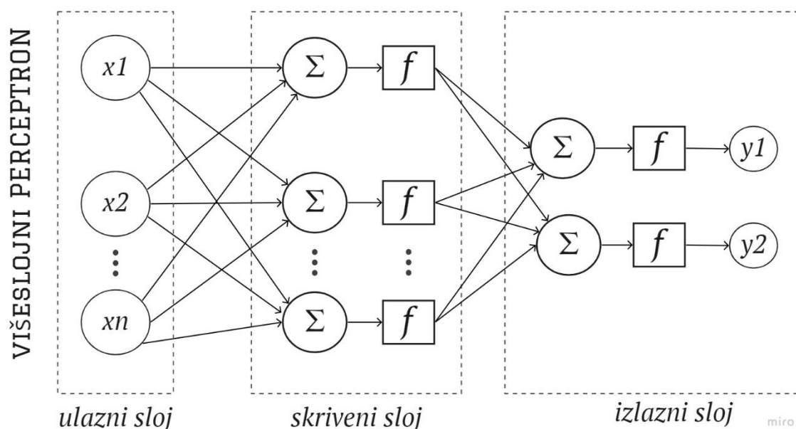
Slika 8 Višeslojni perceptron
